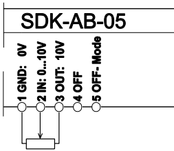
Ansteuerung mit Standardpoti
