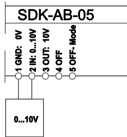
Ansteuerung mit externer Spannungsquelle
