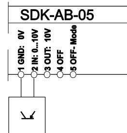
Ansteuerung mit Sinkstromquelle (LV-L2EVG)
