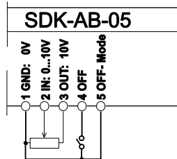
Kontakt offen = Aus Kontakt geschlossen = Ein
