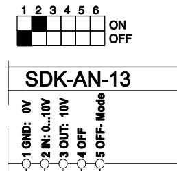
Kontakt offen = Aus Kontakt geschlossen = Ein
