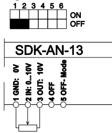
Ansteuerung mit Standardpoti
