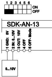
Ansteuerung mit externer Spannungsquelle
