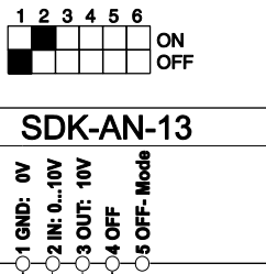
Kontakt offen = Ein Kontakt geschlossen = Aus
