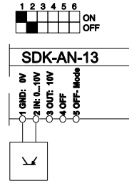
Ansteuerung mit Sinkstromquelle (LV-L2EVG)
